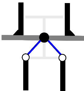
Figuur 4.6 Randcondities van de knoop in het FEA-model.
