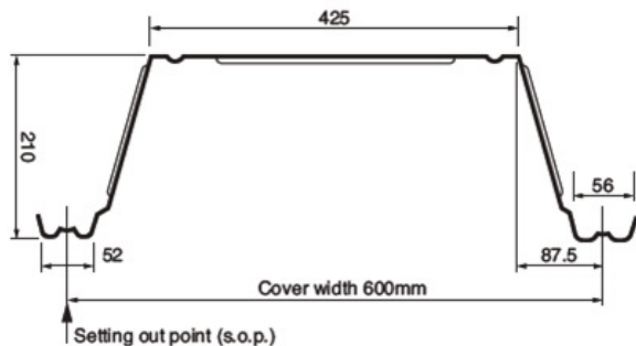
Figuur 4.2 Het profiel van de stalen plaat in de Comflor 210 vloer.
