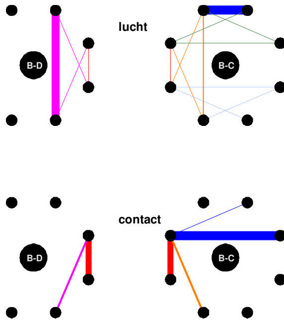
Figuur 4.3 Visualisatie van de geluidisolatie per pad.
