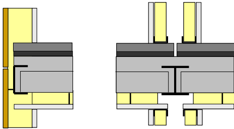
Figuur 4.1 Systeem 1b, staalskeletbouw met een hoge staalplaatbetonvloer.
