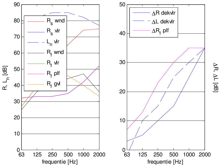
Figuur 4.5 Isolatiewaarden van de aangrenzende onderdelen.
