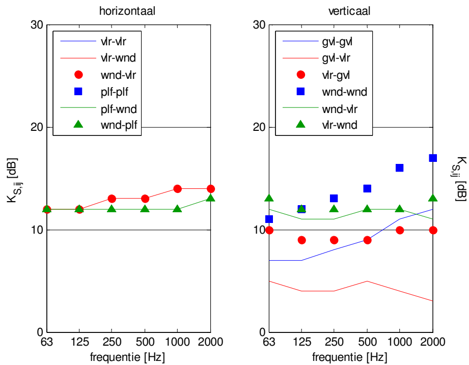
Figuur 4.4 Trillingoverdrachtverzwakking van de knoop voor elk pad.
