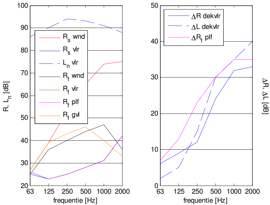
Figure 23 Isolatiewaarden van de aangrenzende onderdelen.
