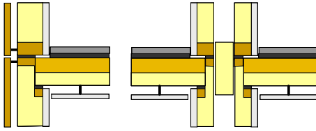
Figuur 19 Systeem 2b, het Maskeradesysteem.
