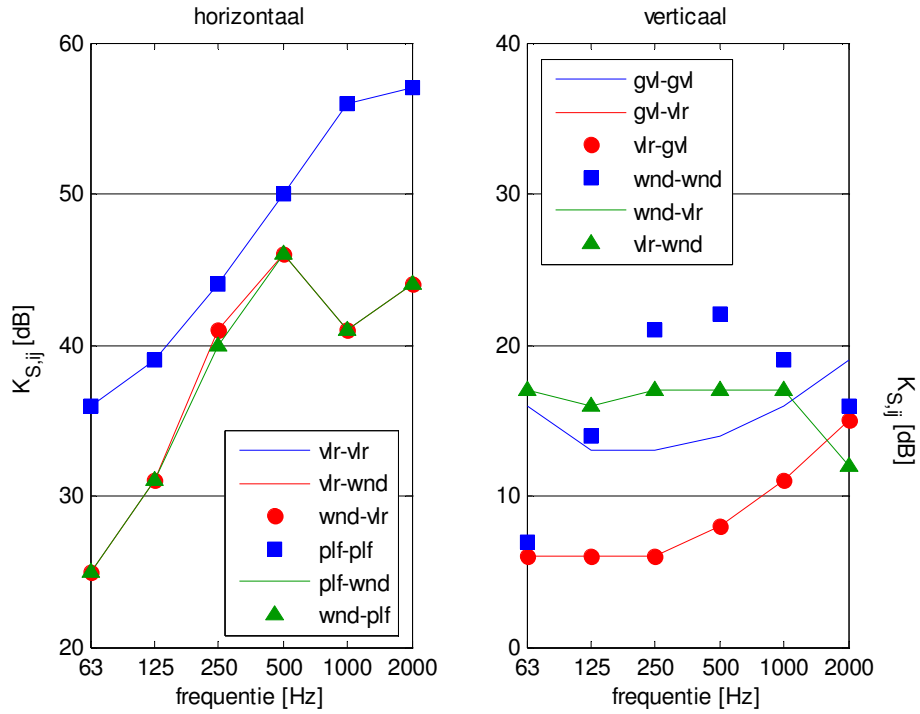
Figure 22 Trillingoverdrachtverzwakking van de knoop voor elk pad.
